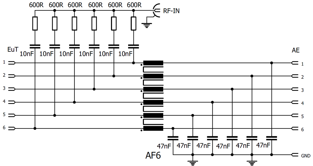
Bild 3: Prinzipschaltbild CDN AF6 Fig. 3: principal circuitry CDN AF6
