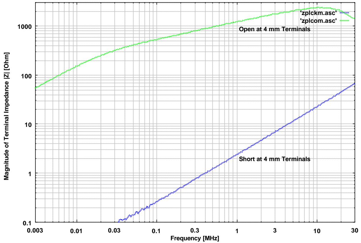
Betrag der Klemmenimpedanz bei Leerlauf und Kurzschluß
