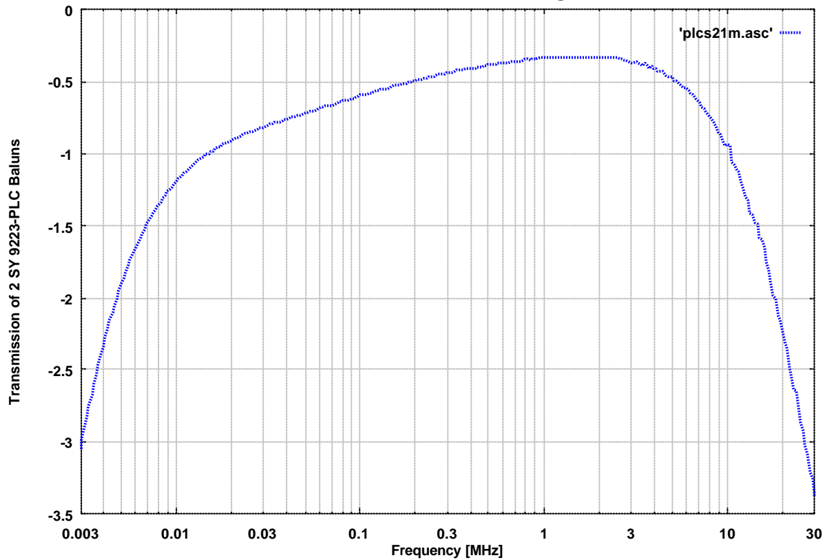
Transmission von 2 SY 9223-Übertragern
