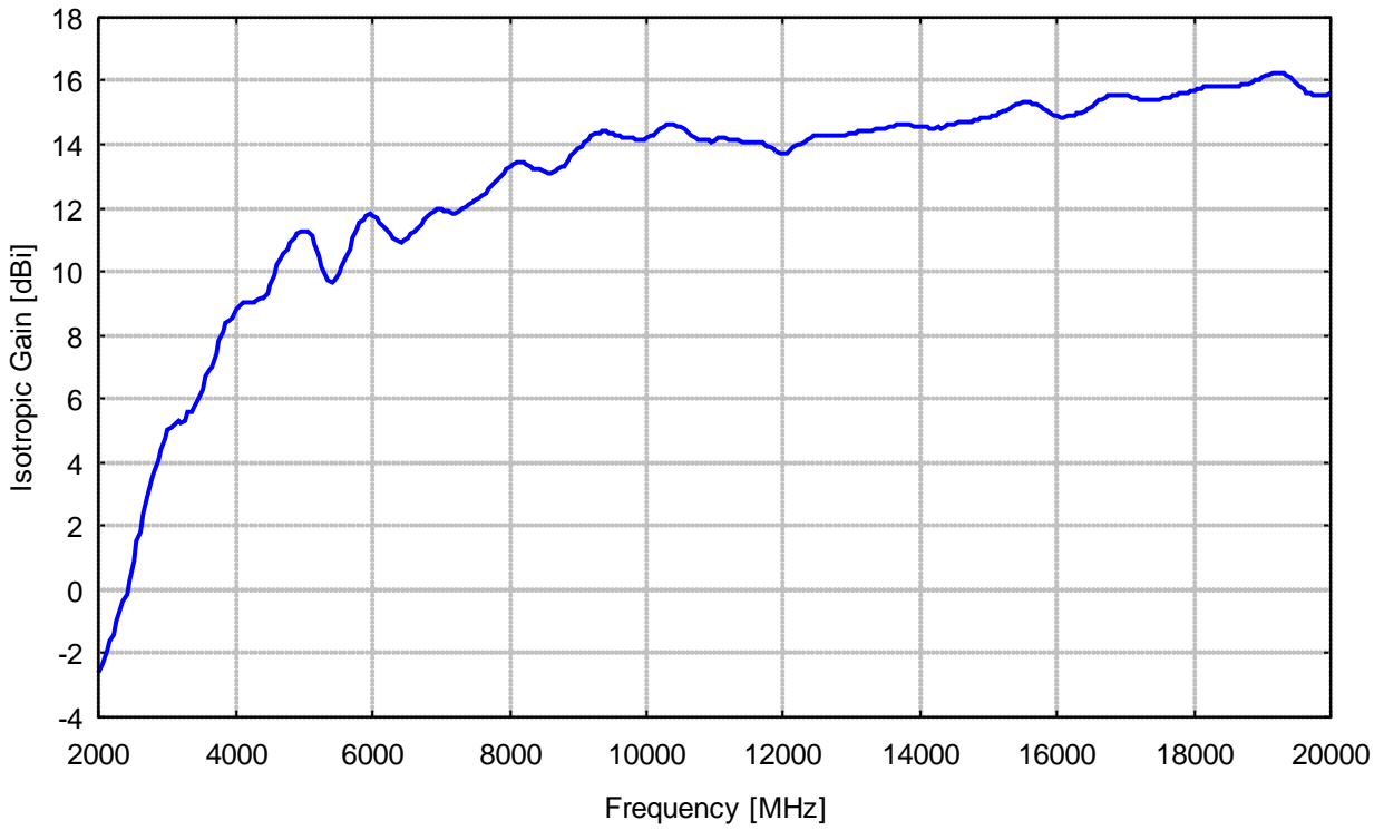
Isotropgewinn
