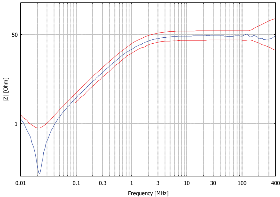
Abb. 3: Betrag der Impedanz an den Prüflingsklemmen nach DO-160 (Kalibrieradapter KA 8125 erforderlich), BNC mit 50 \Omega Abschluss.
